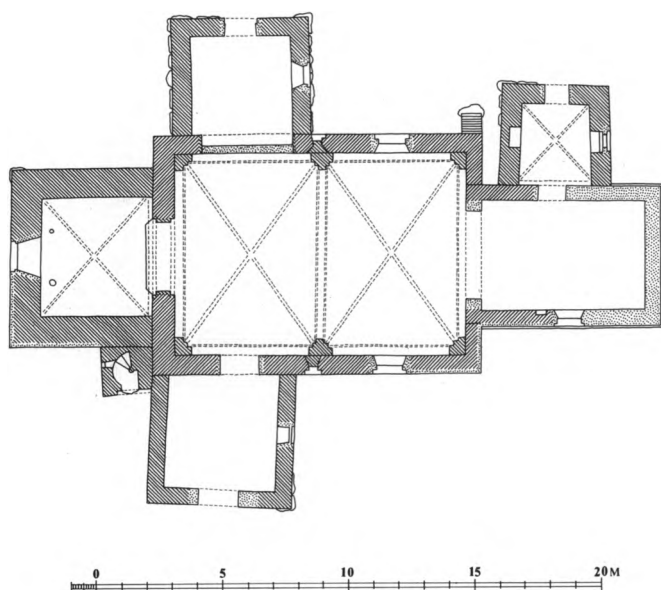
Fig. 5. Plan. 1:300. Målt af C. G. Schultz 1929, revideret af HJ 1981 og tegnet af Marianne Nielsen 1990. Signaturforklaring s. 9. - Ground-plan. Key on p. 9.
